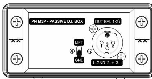
FIG. 2 - Painel Traseiro
